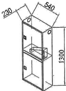
Рис. 1 Шкаф навесной закрытый правый с еврозамком
