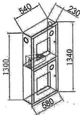
Рис. 2 Шкаф встроенный открытый левый
